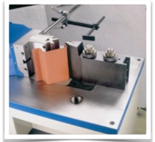
Multi-Vee Press Brake
